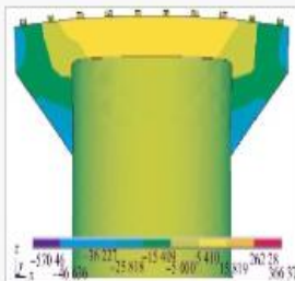
预应力加固后主应力云图
