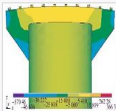
预应力加固后主应力云图
